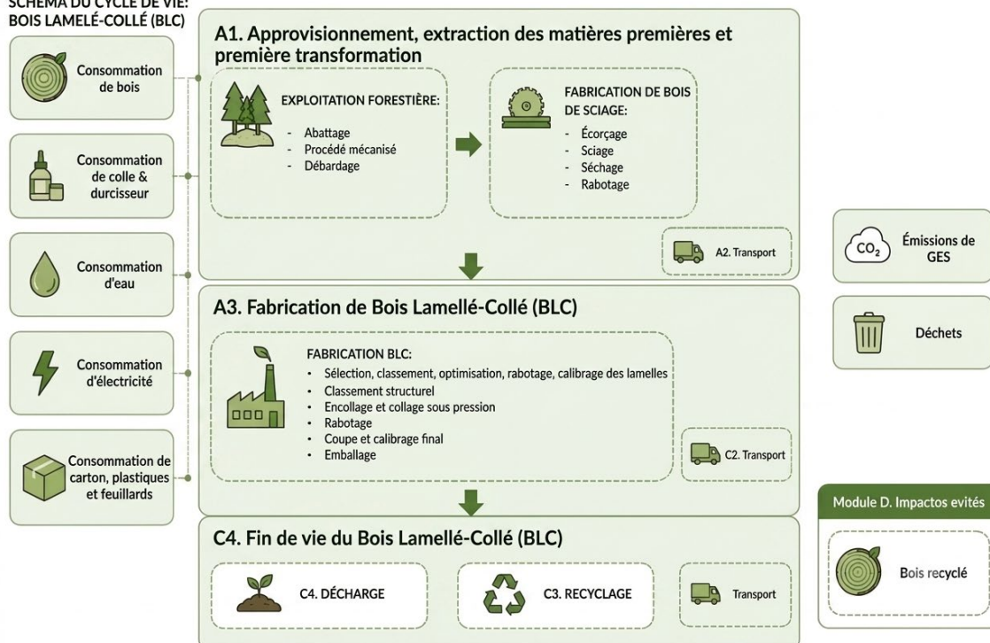
SCHÉMA DU CYCLE DE VIE: BOIS LAMELÉ-COLLÉ (BLC)
