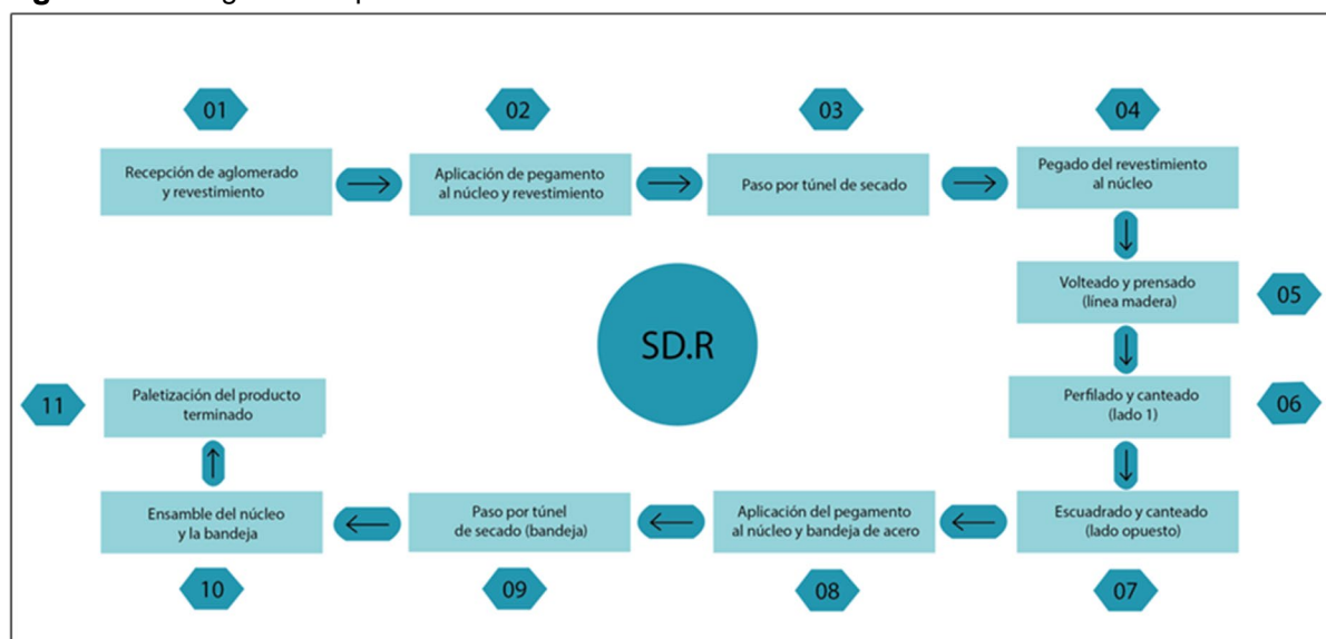
Figura 3-1. Diagrama de procesos.
