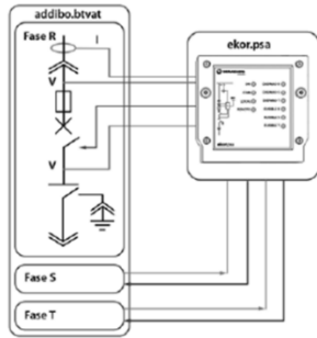
Envolvente tripolar con relé ekor.psa
