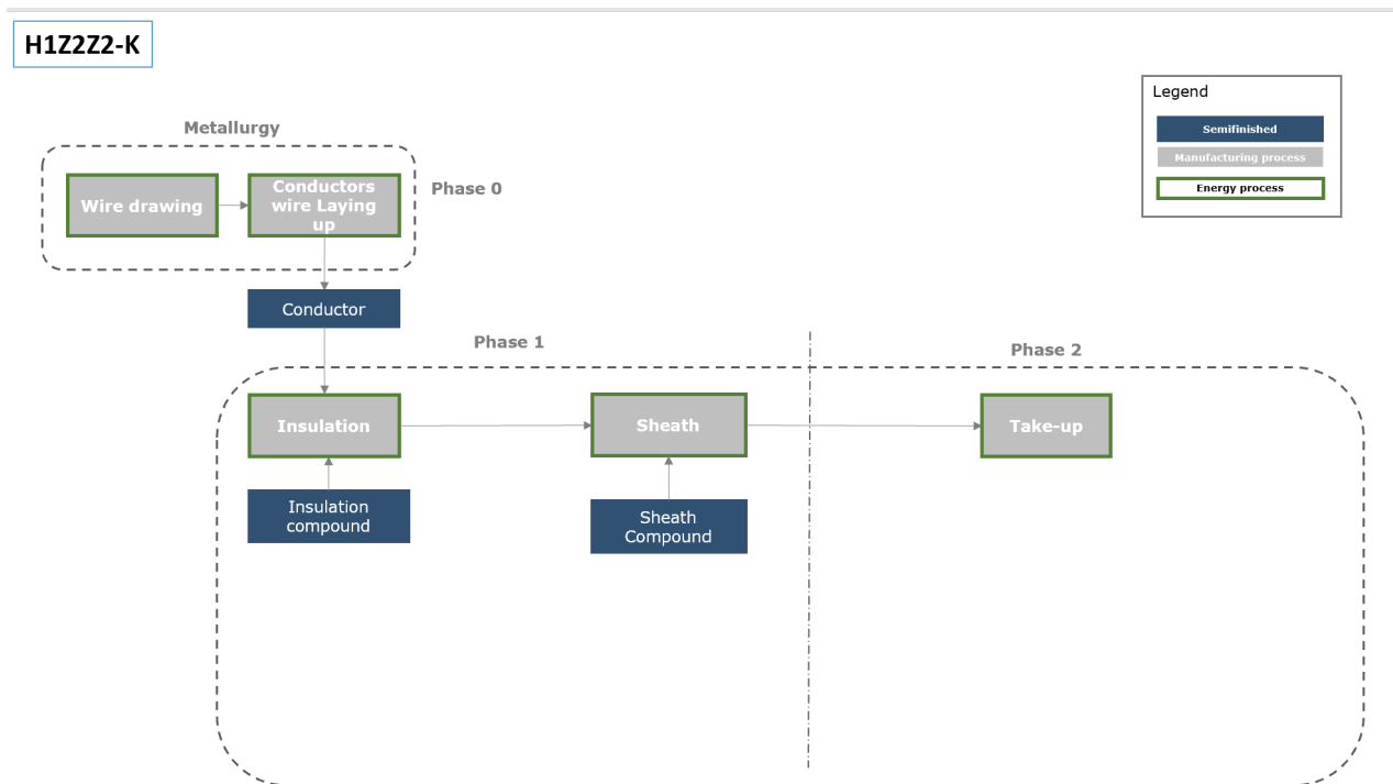
Diagrama de flujo del proceso de fabricación
