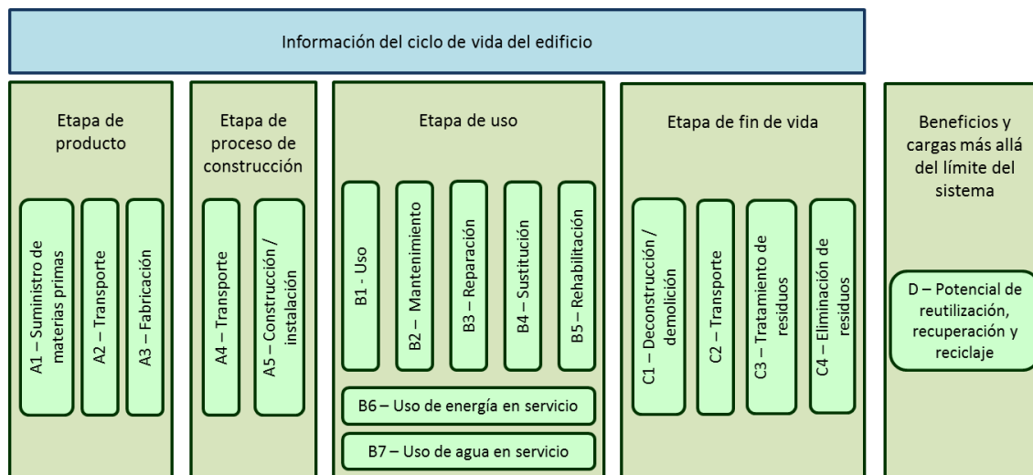
Figura AA – Módulos de información para la evaluación de edificios
