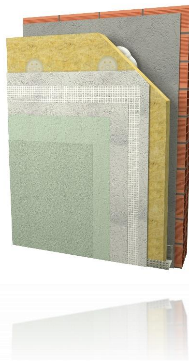
Figura 1. Componentes de un SATE (fuente: Artículos Técnicos SATE, ANFAPA (septiembre, 2020))
